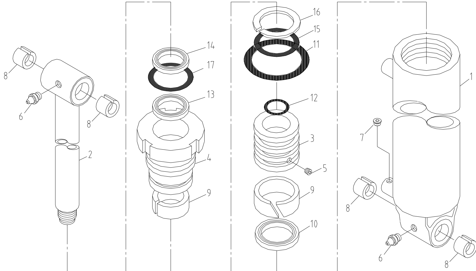
데릭 실린더 조립체 Fig. 2-2 SCS2016 DERRICK CYL' ASS'Y
