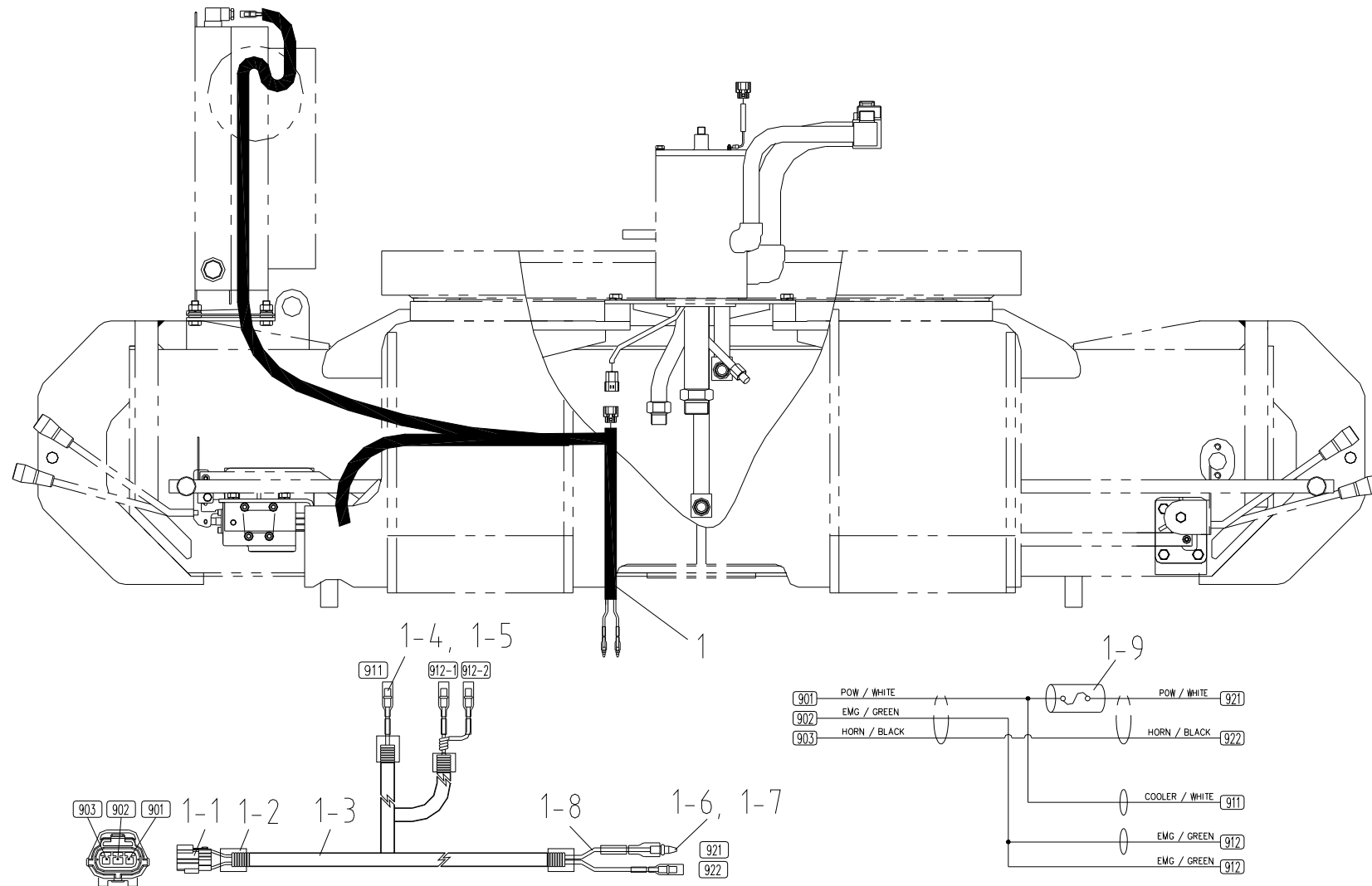
프레임 전선 Fig. 17-1-1 SCS2016 FRAME WIRING
