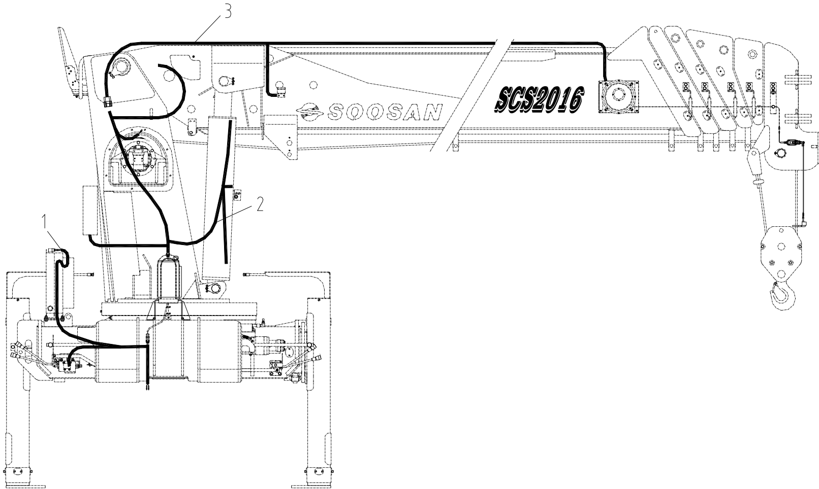
과하중방지장치 전선 조립체 Fig. 17-1 SCS2016 AML WIRING ASS'Y
