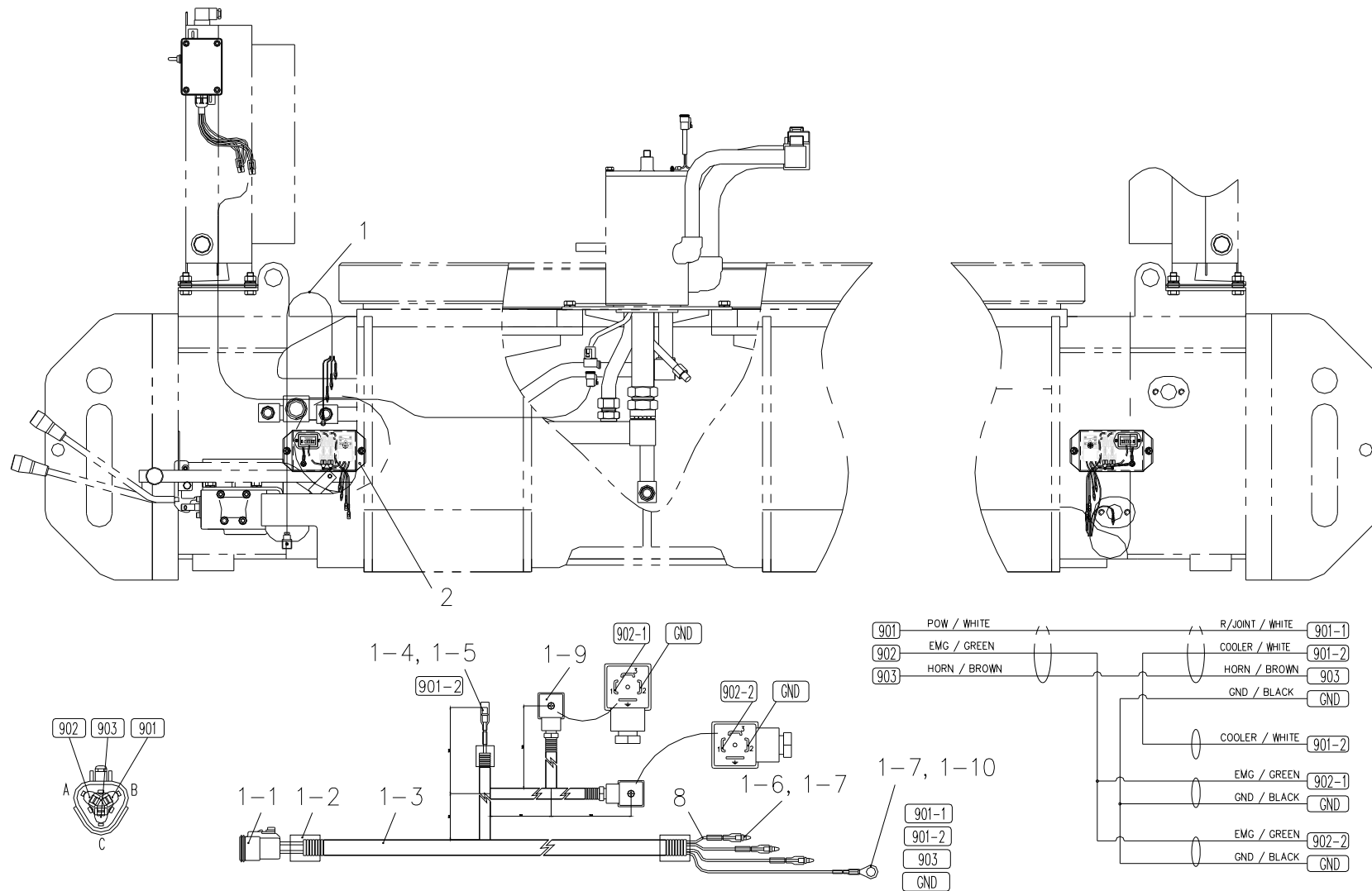
프레임 전선 Fig. 10-1 SCS2016 FRAME WIRING
