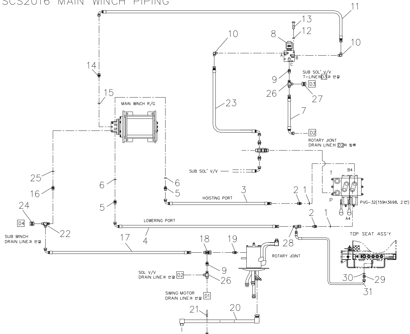
메인 윈치 배관 Fig. 5-5 SCS2016 MAIN WINCH PIPING
