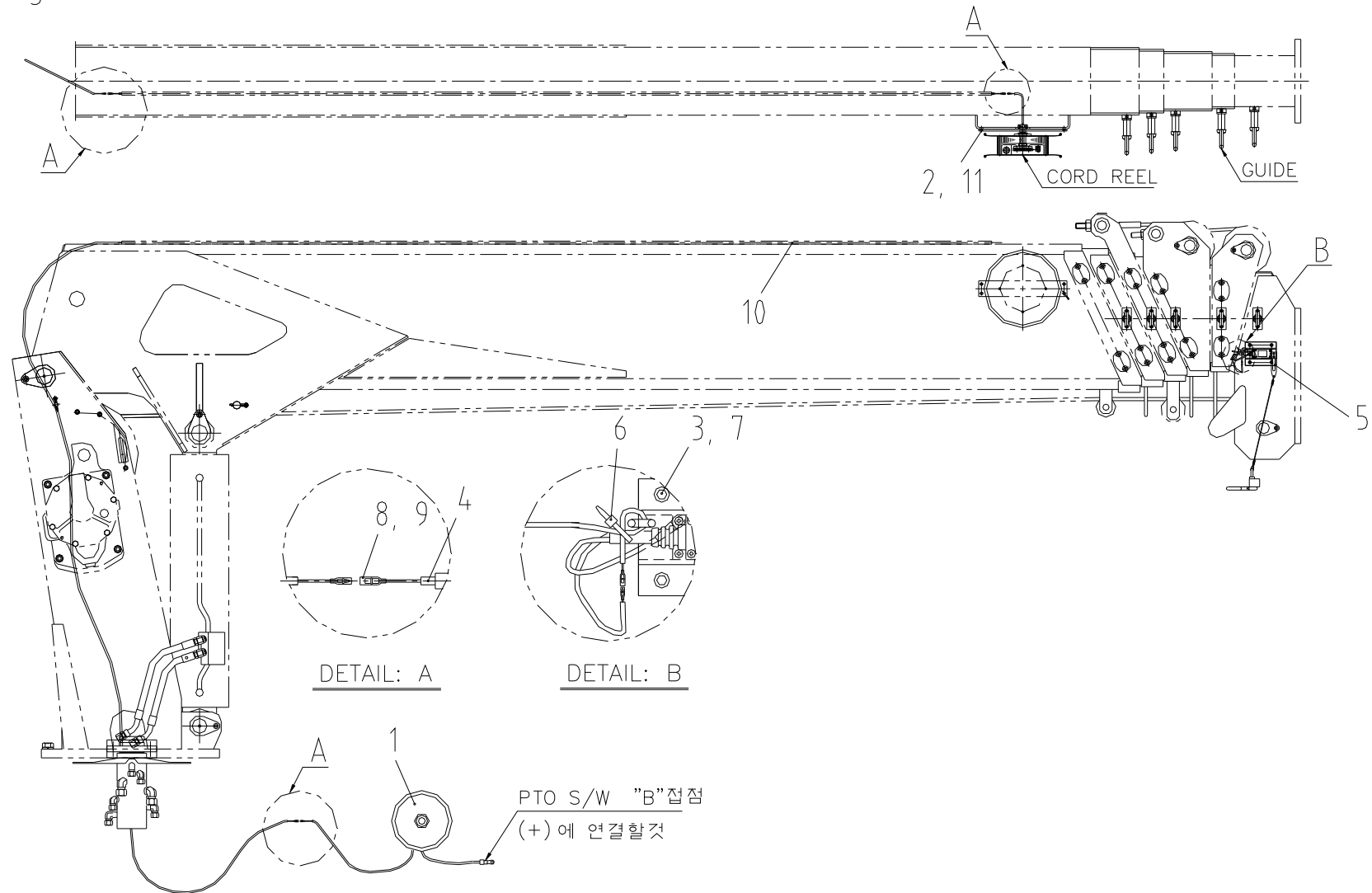
Fig. 16 SCS2016 과권방지장치 조립체
