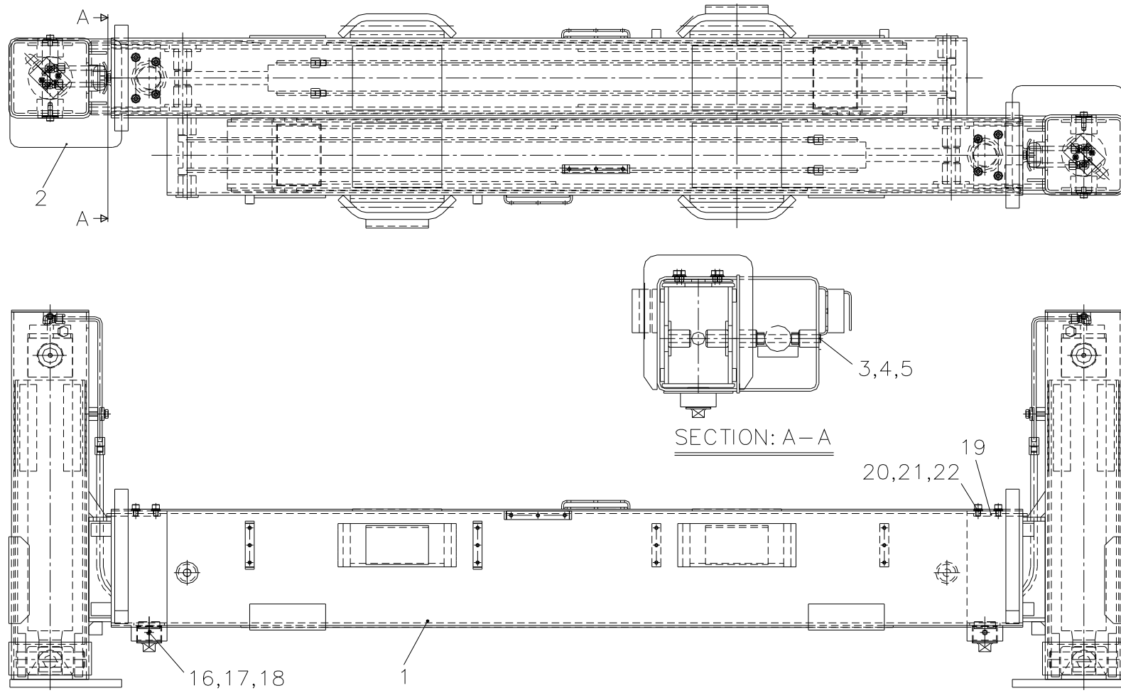
후방 아우트리거 조립체 Fig. 9-1-1 SCS2016 REAR OUTRIGGER ASS'Y
