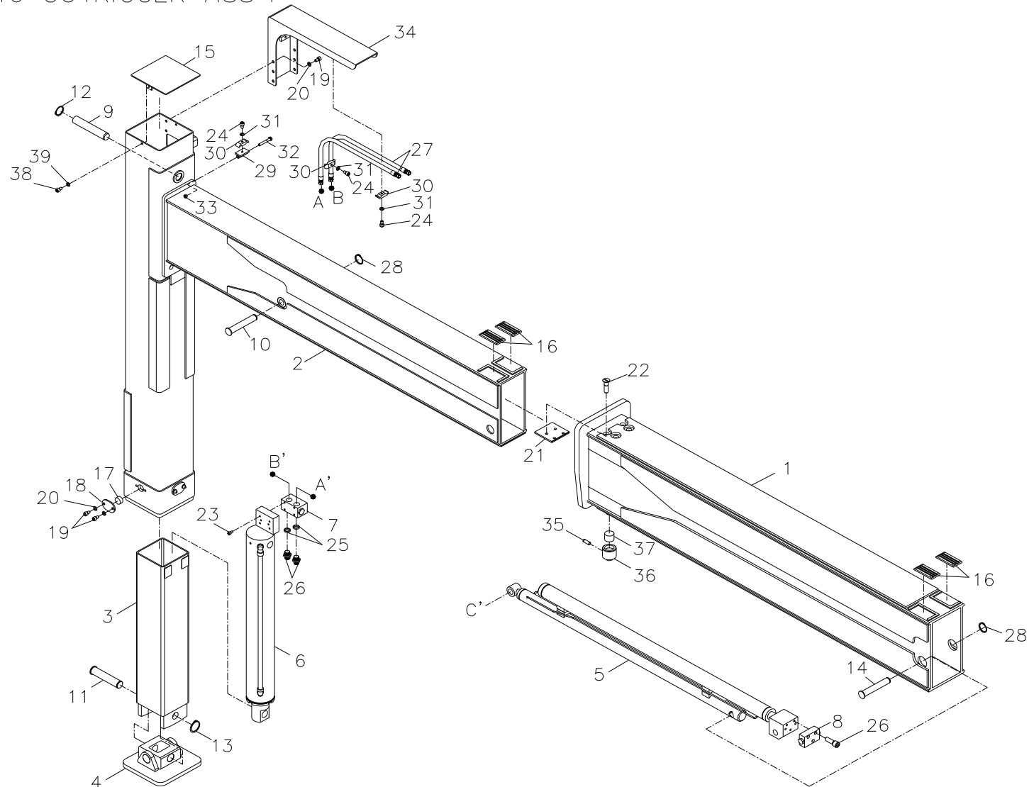
아우트리거 조립체 Fig. 4 SCS2016 OUTRIGGER ASS'Y
