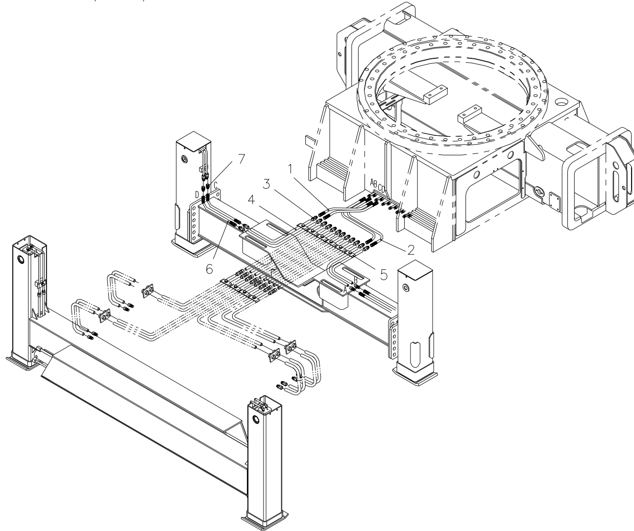
중간 아웃리거 장착 배관 파트 Fig. 15 SCS2016 M/O M/T PIPING PART
