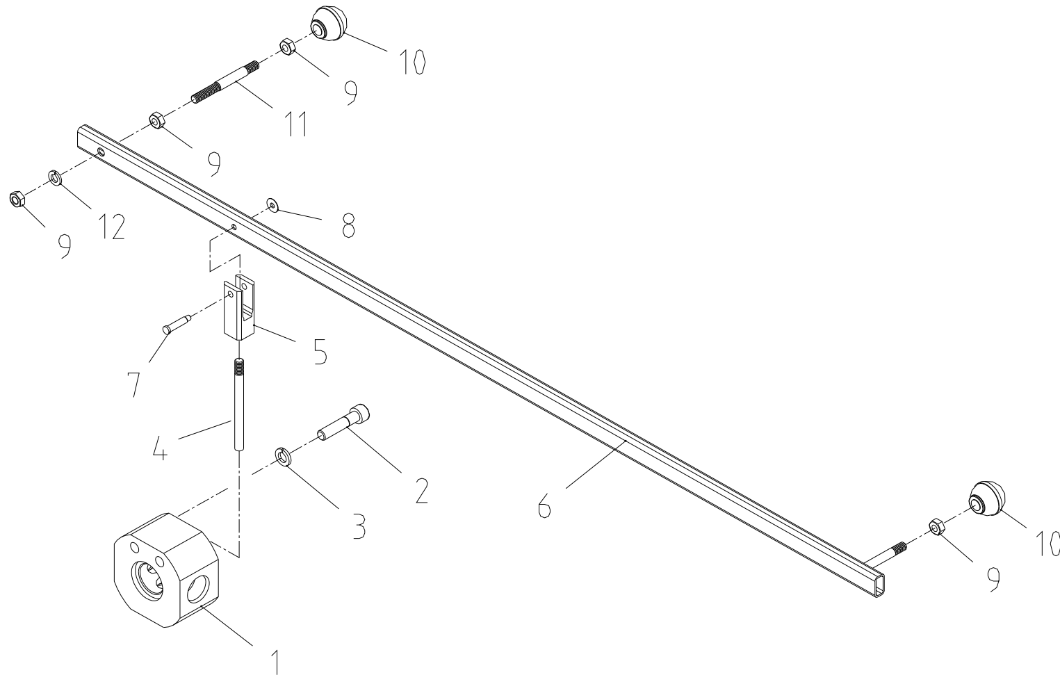
디버터 밸브 셋트 Fig. 3-3 SCS2016 DIVERTER V/V SET
