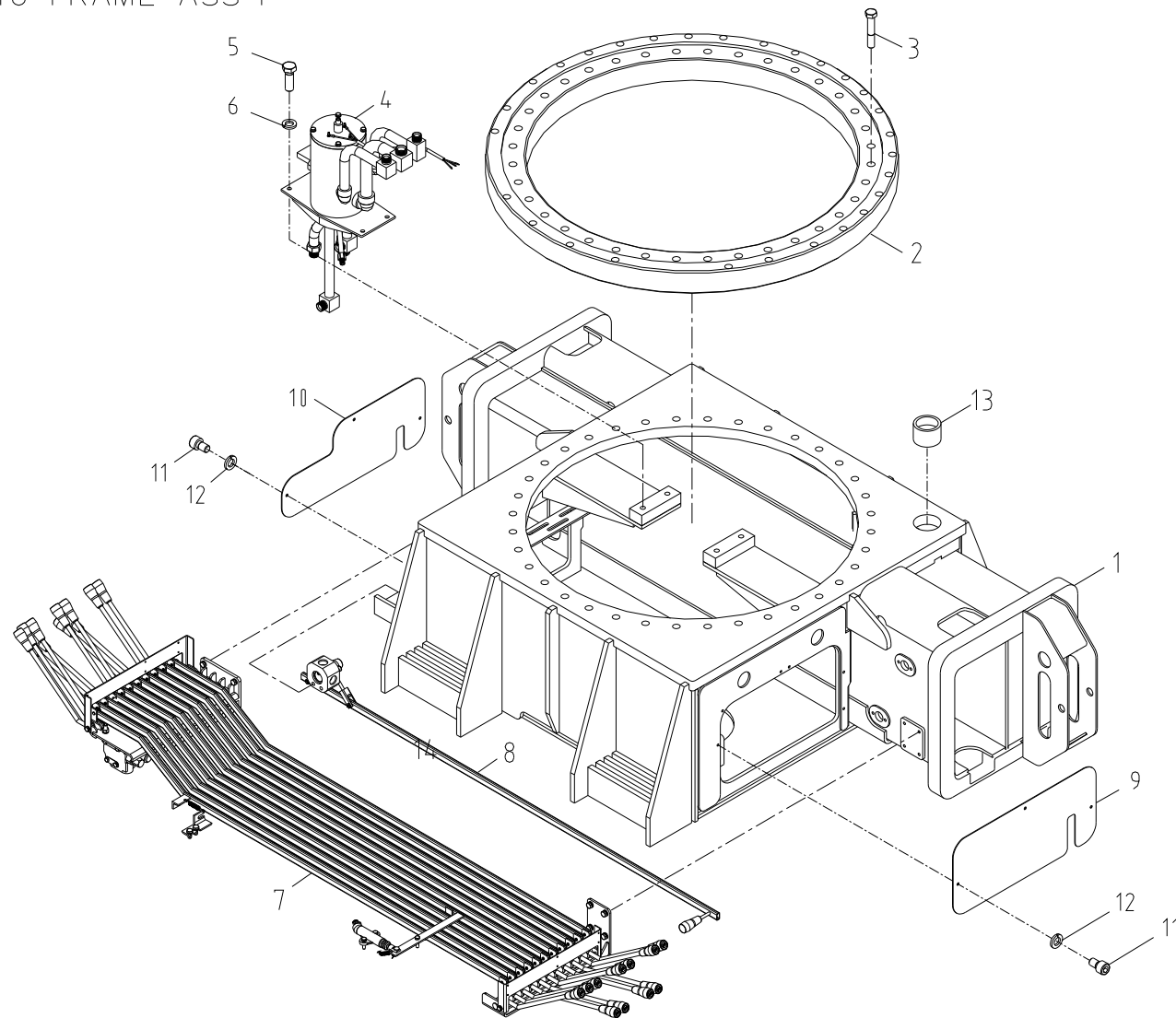
프레임 조립체 Fig. 3 SCS2016 FRAME ASS'Y
