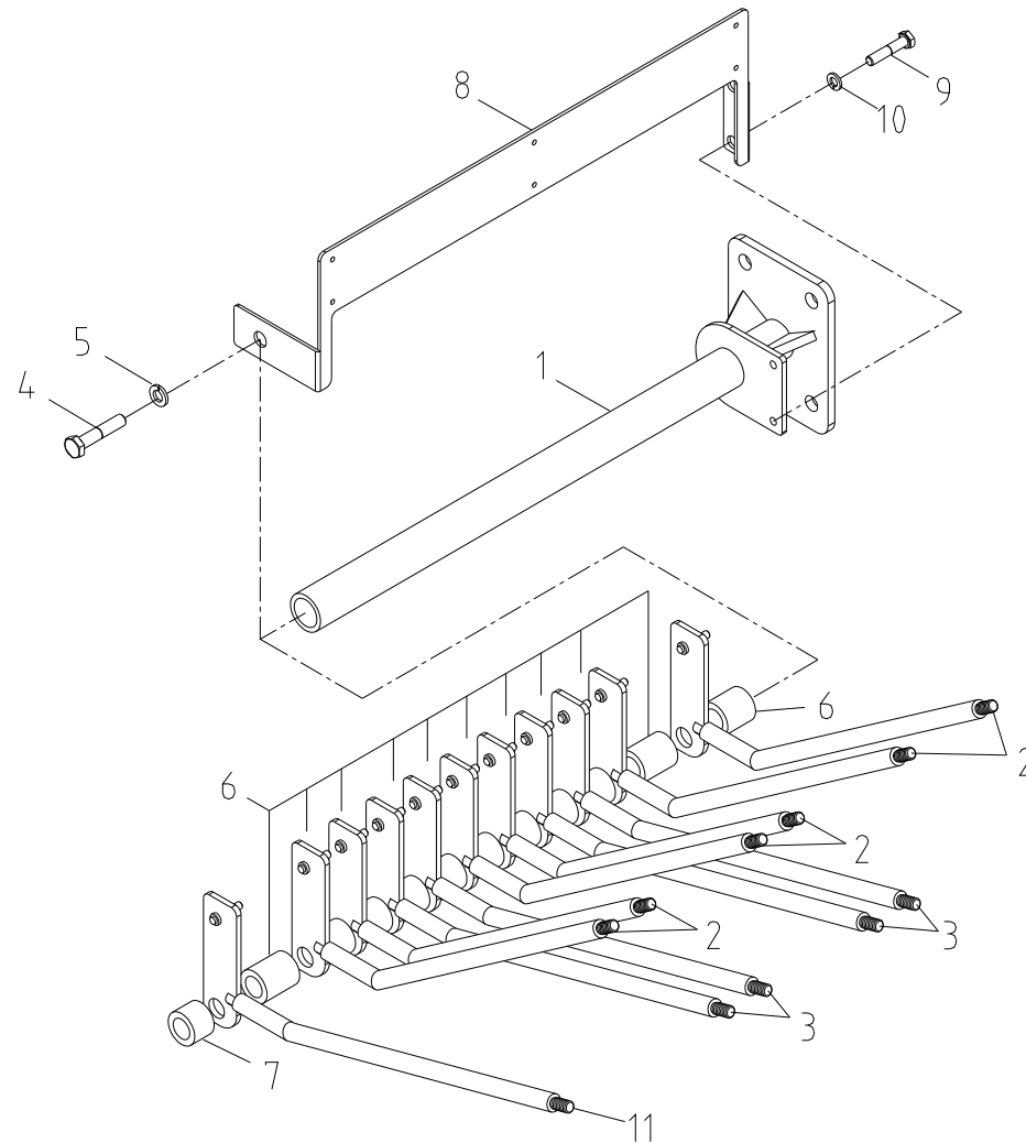
레버 스텐드 셋 Fig. 3-2-2 SCS2016 LEVER STAND SET
