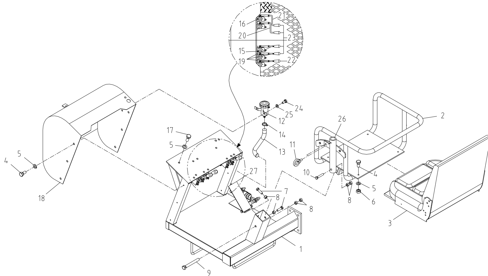
탑 시트 조립체 Fig. 6 SCS2016 TOP SEAT ASS'Y
