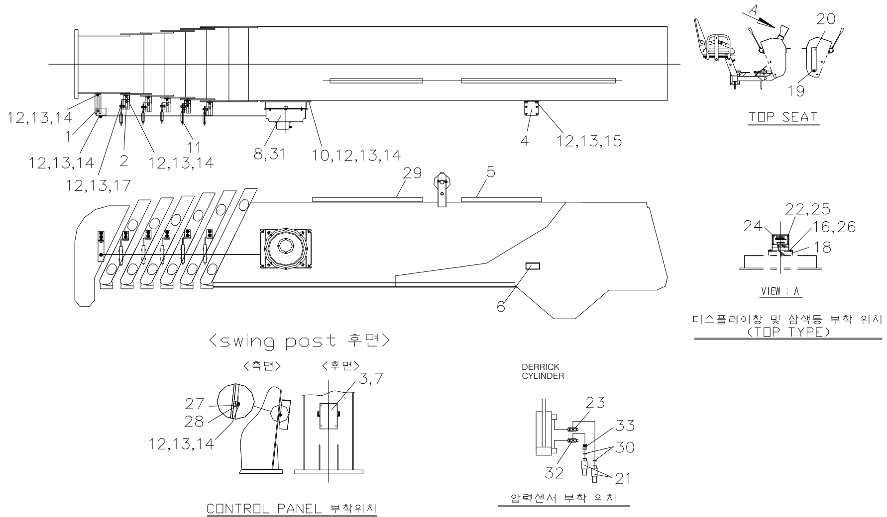
Fig. 17 SCS2016 과하중방지장치 설치도
