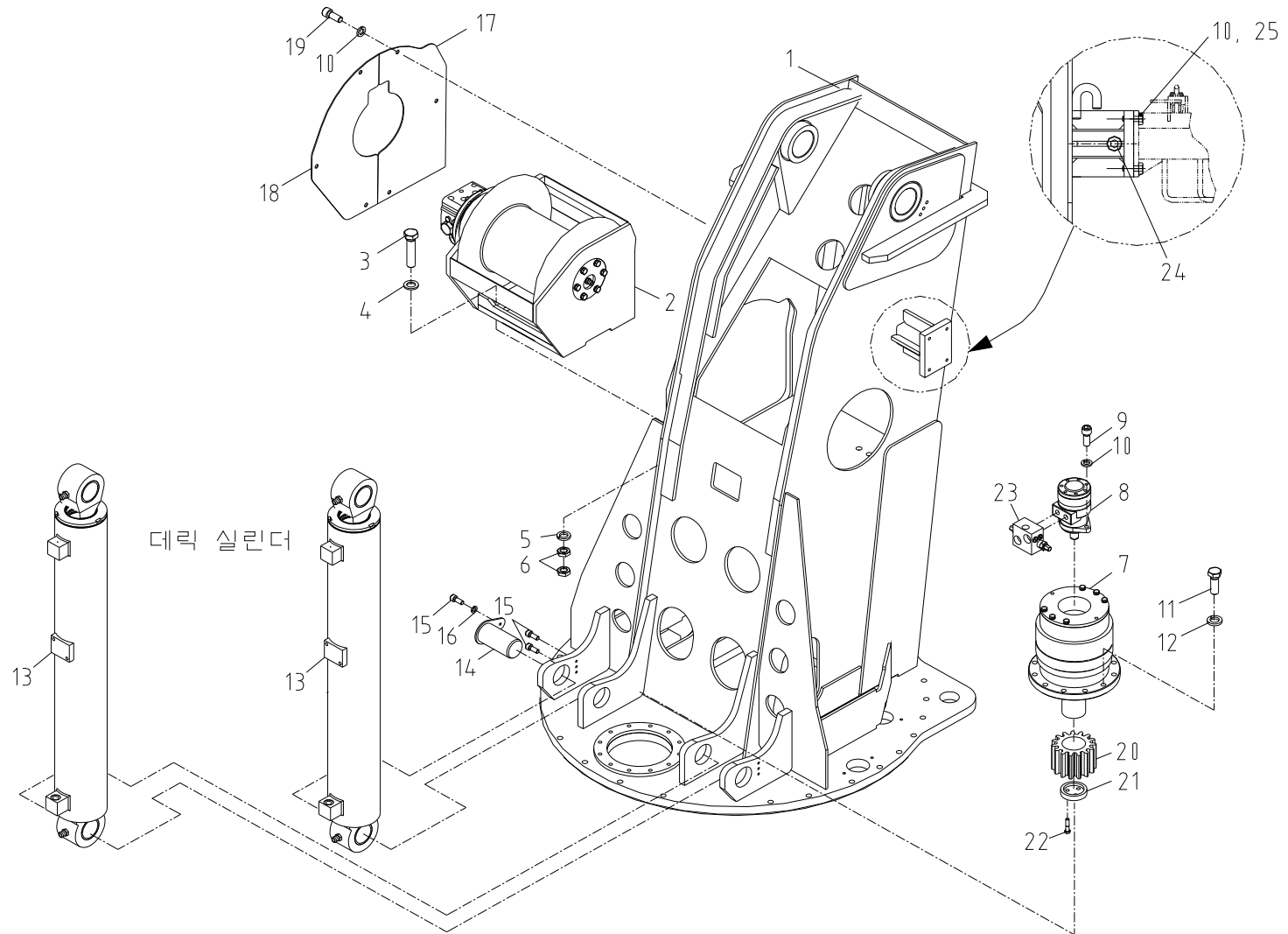
스윙 포스트 조립체 Fig. 2 SCS2016 SWING POST ASS'Y
