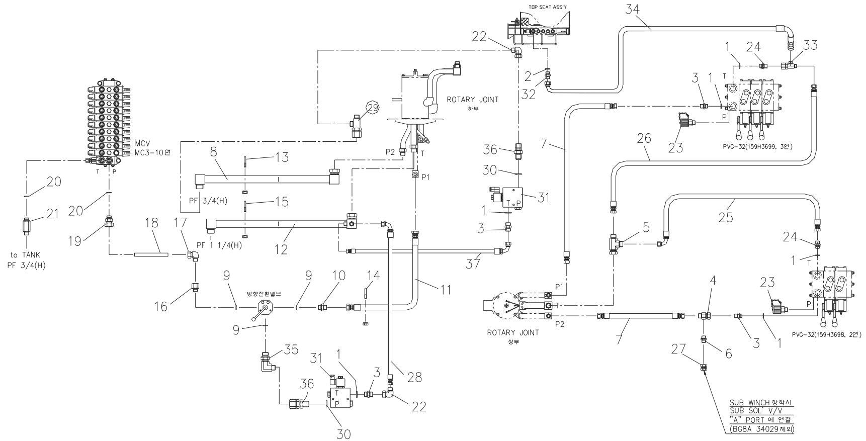
디스트리뷰터 배관 Fig. 5-1 SCS2016 DISTRIBUTOR PIPING
