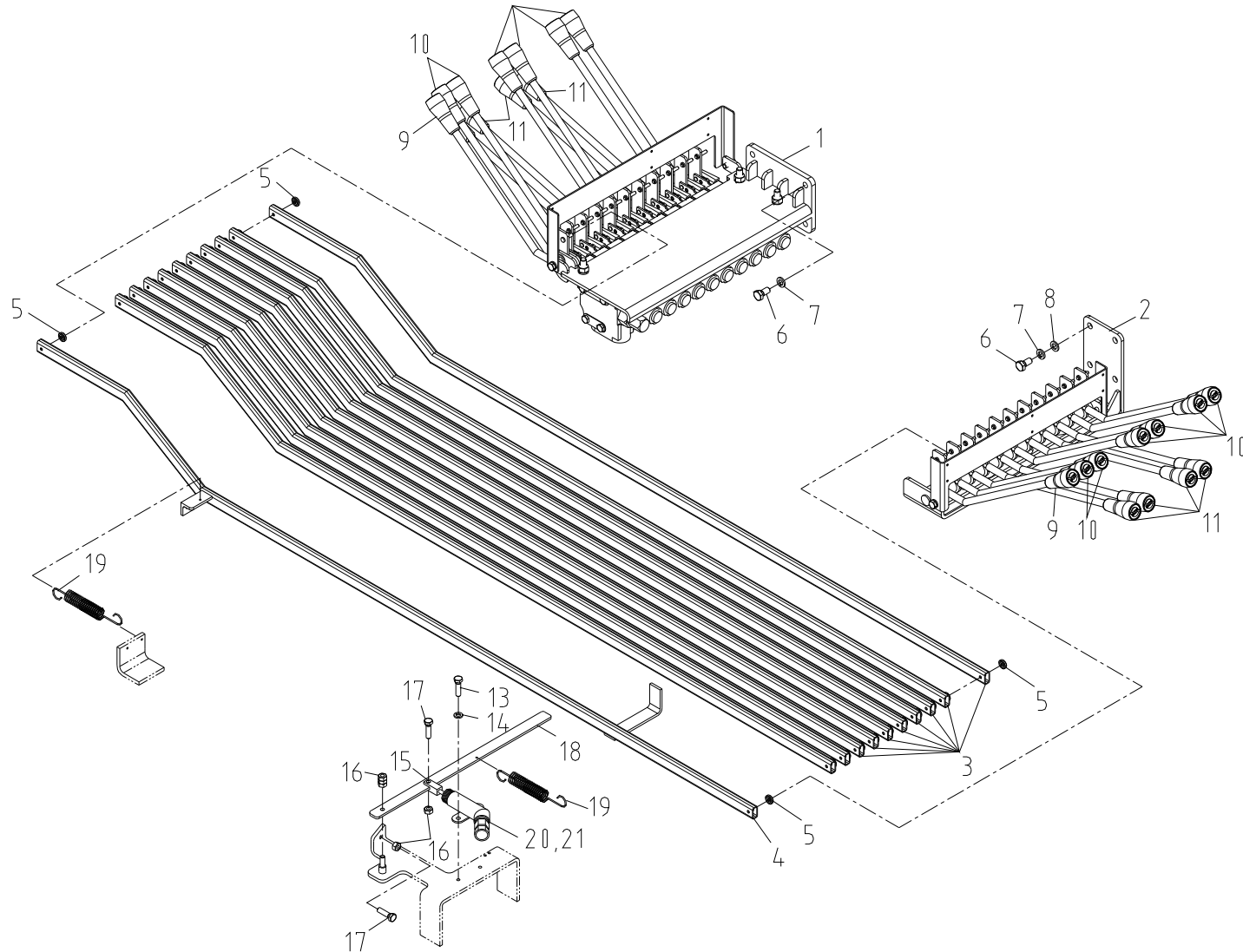
오퍼레이션 조립체 Fig. 3-2 SCS2016 OPERATION ASS'Y 10
