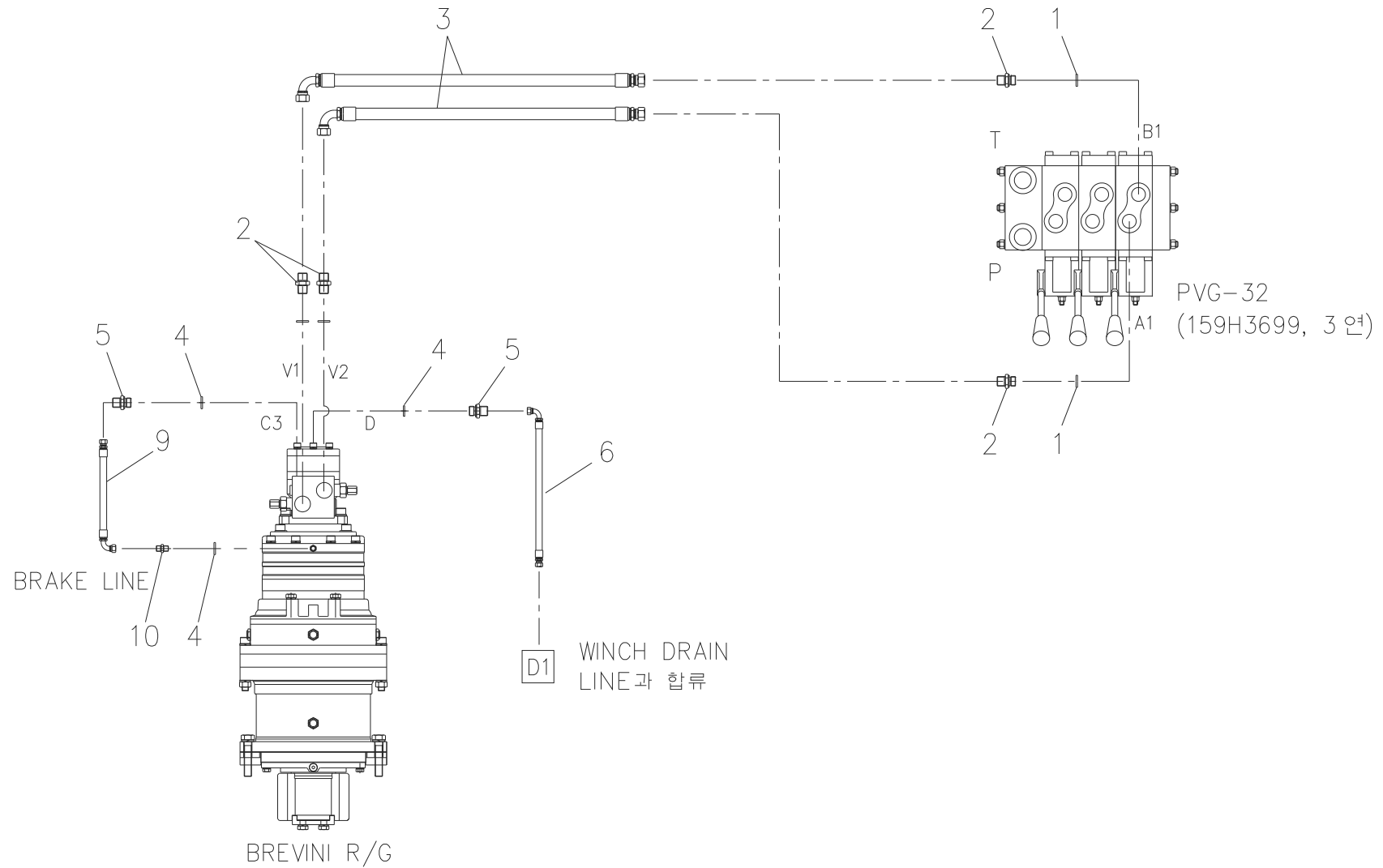
스윙 배관 Fig. 5-2 SCS2016 SWING PIPING
